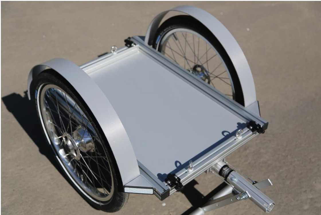
ROBERT mit Schutzblechen und Federriegeln zur Aufnahme einer Faltbox
